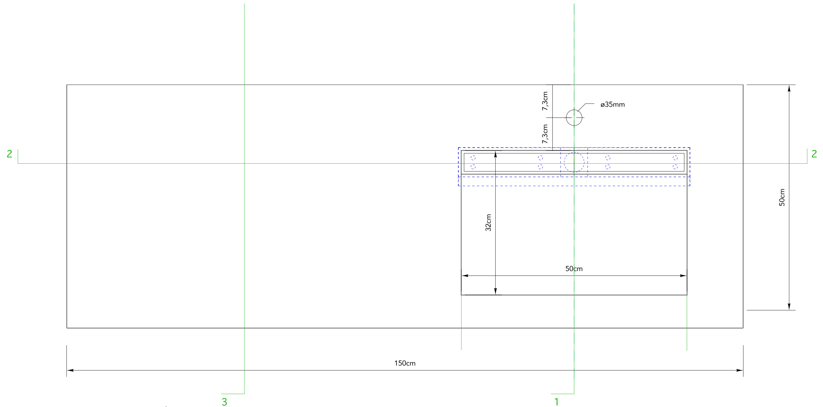
VISTA DALL'ALTO, scala 1:5
