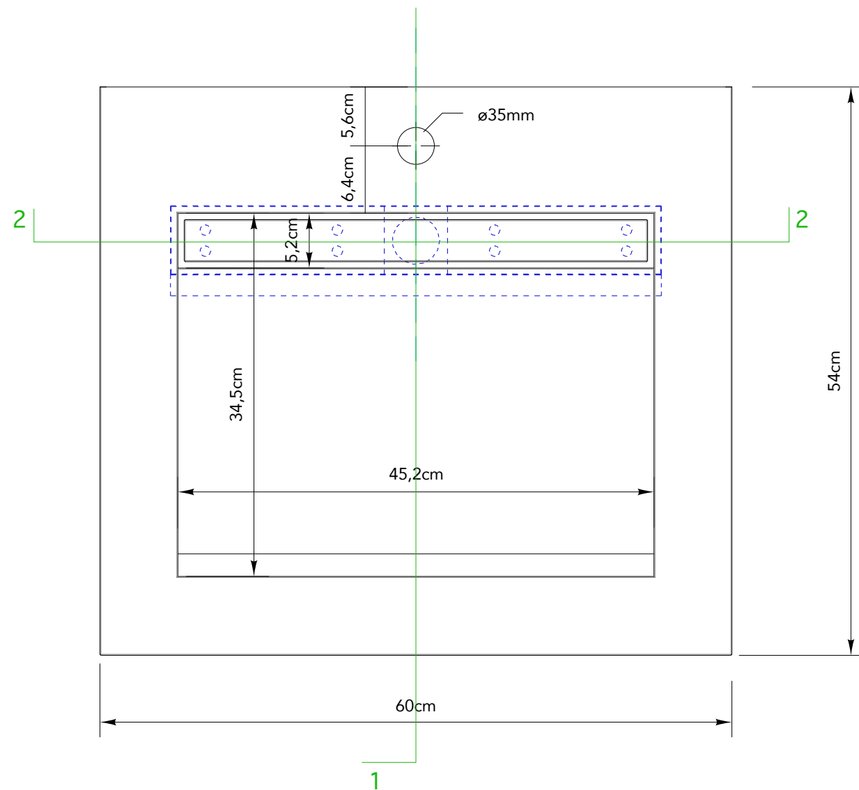
VISTA DALL'ALTO, scala 1:5
